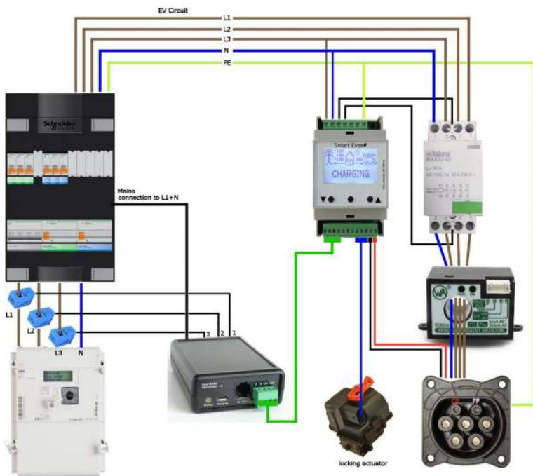
Prinzip Schema Wallbox mit SmartEVSE
